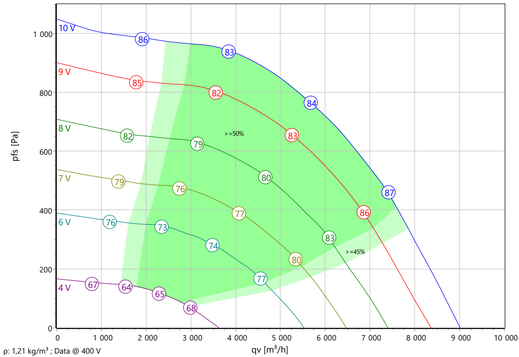
p: 1,21 kg/m³ ; Data @ 400 V
